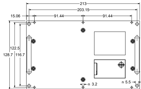
Stecker hinten
