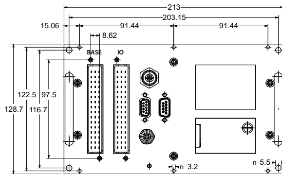
Stecker vorne
